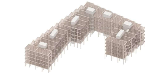
Konstruktive Darstellung der überlappenden Tragwerke
